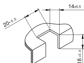
Монтажное отверстие
