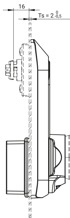
Исполнение для колпачка [N]
