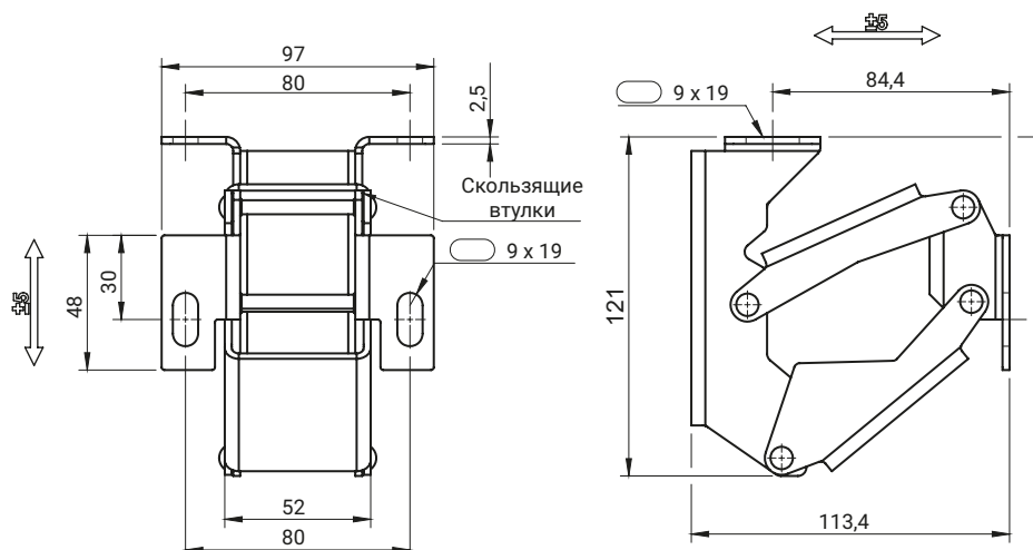
позиция закрытая
