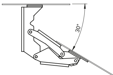
позиция открытая
