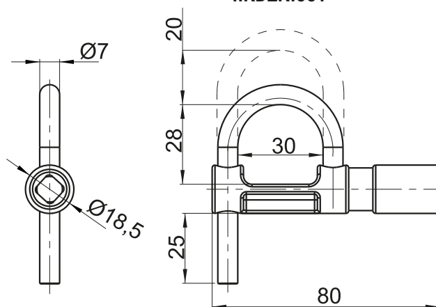
НАВЕСНОЙ ЗАМОК SN 4.KDZN.001
