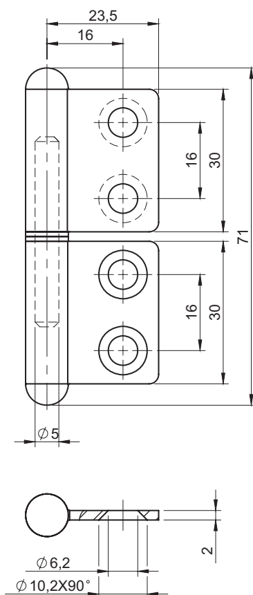
ПЕТЛЯ ЛЕВАЯ 3.ST127.003SN - B
