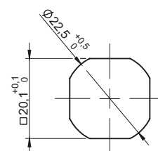
Размер монтажного отверстия
