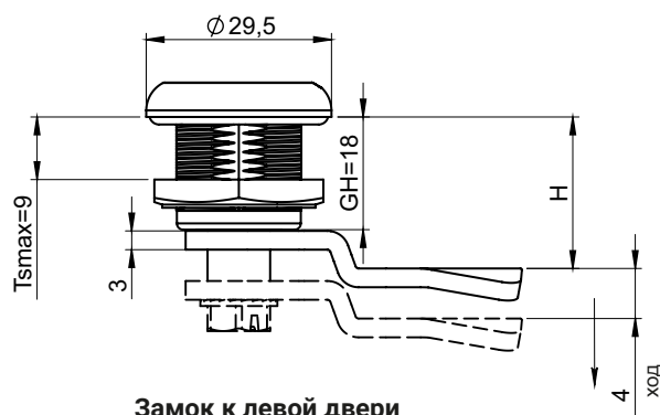
Замок к левой двери
