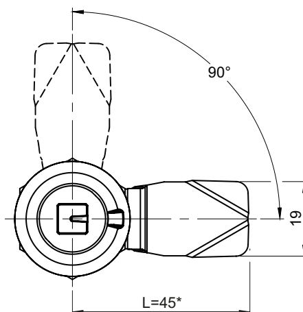
Замок к левой двери
